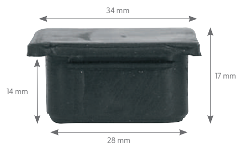
I TR000315 Bouchon angle caoutchouc.
