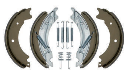
1FK7172 Kit mâchoires 203 x 40 pour 203216-47.
