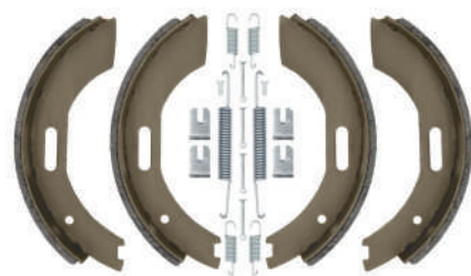
1FK7165 Kit mâchoires 200 x 50 pour S2005-7RASK.
